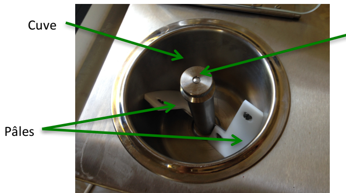
Photo 2 : cuve
